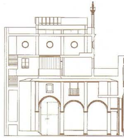
sección.S.6
